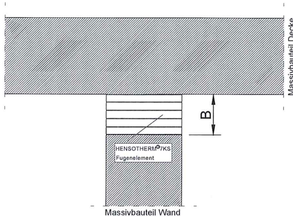
Bild 2 Ausrichtung des „HENSOTHERM® 7KS“ Fugenelementes im Anschlussbereich Wand / Decke
