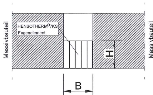
Bild 1 Prinzipskizze zur Anordnung des „ HENSOTHERM® 7KS “ Fugenelementes im Massivbauteil (Decke)
